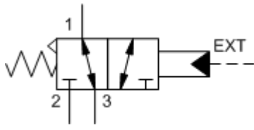
C-Spool
