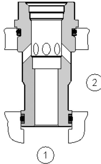
Einschraubbohrungs-Adapter von SUN T-16A auf SUN T-13A.
