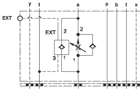
Meter out A
